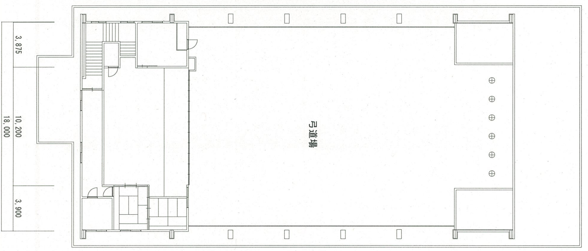
2階平面図
