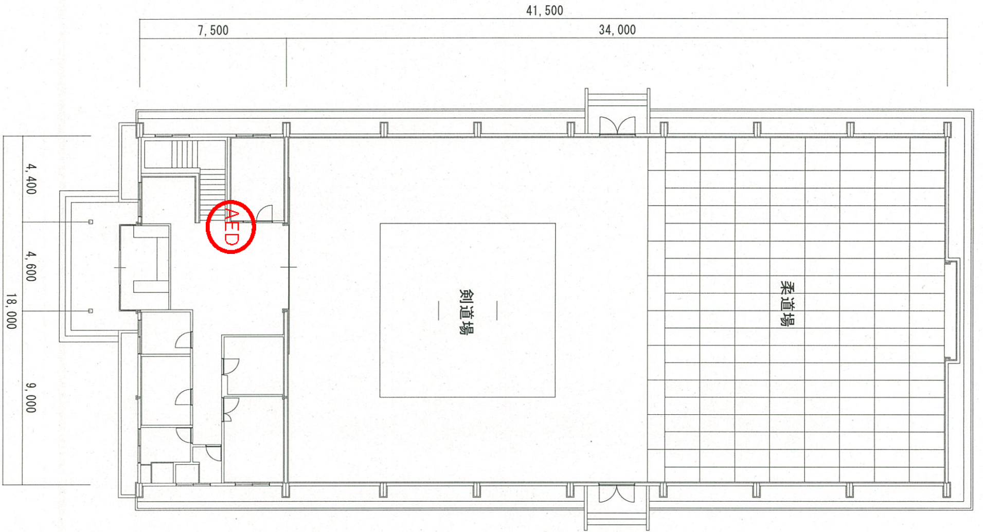
1階平面図
