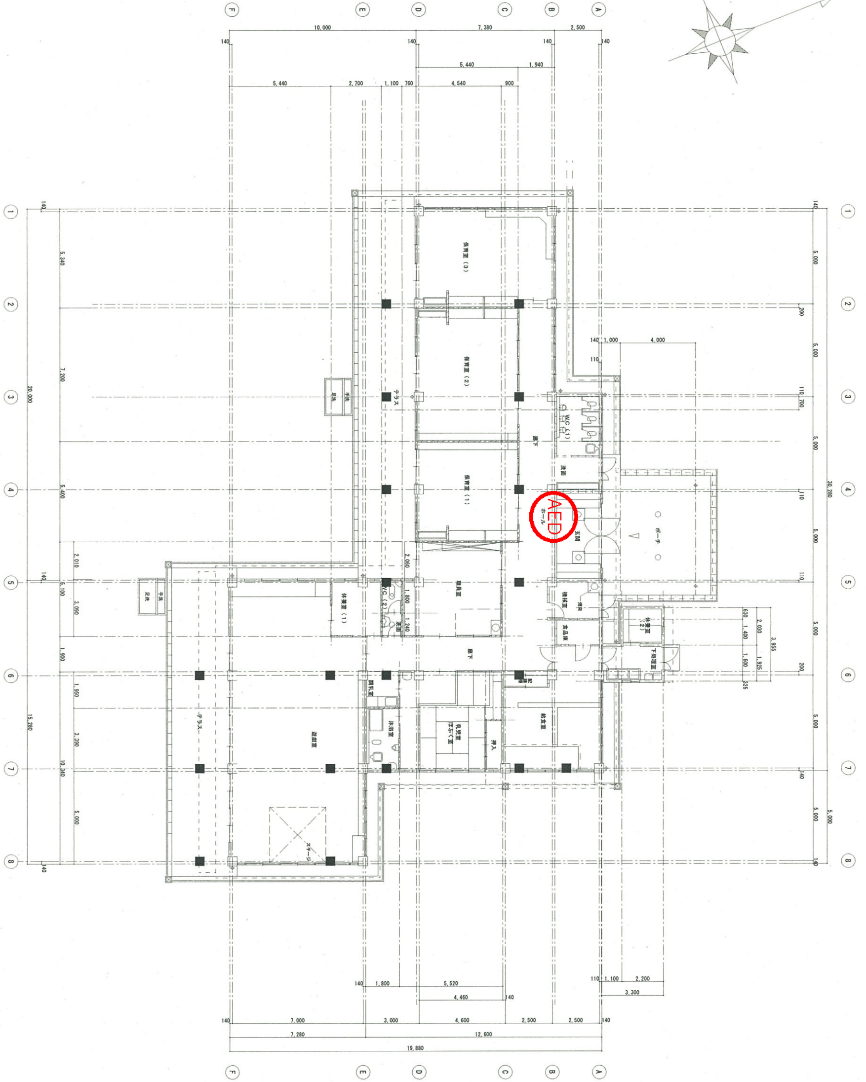
平面図 S=1/100
