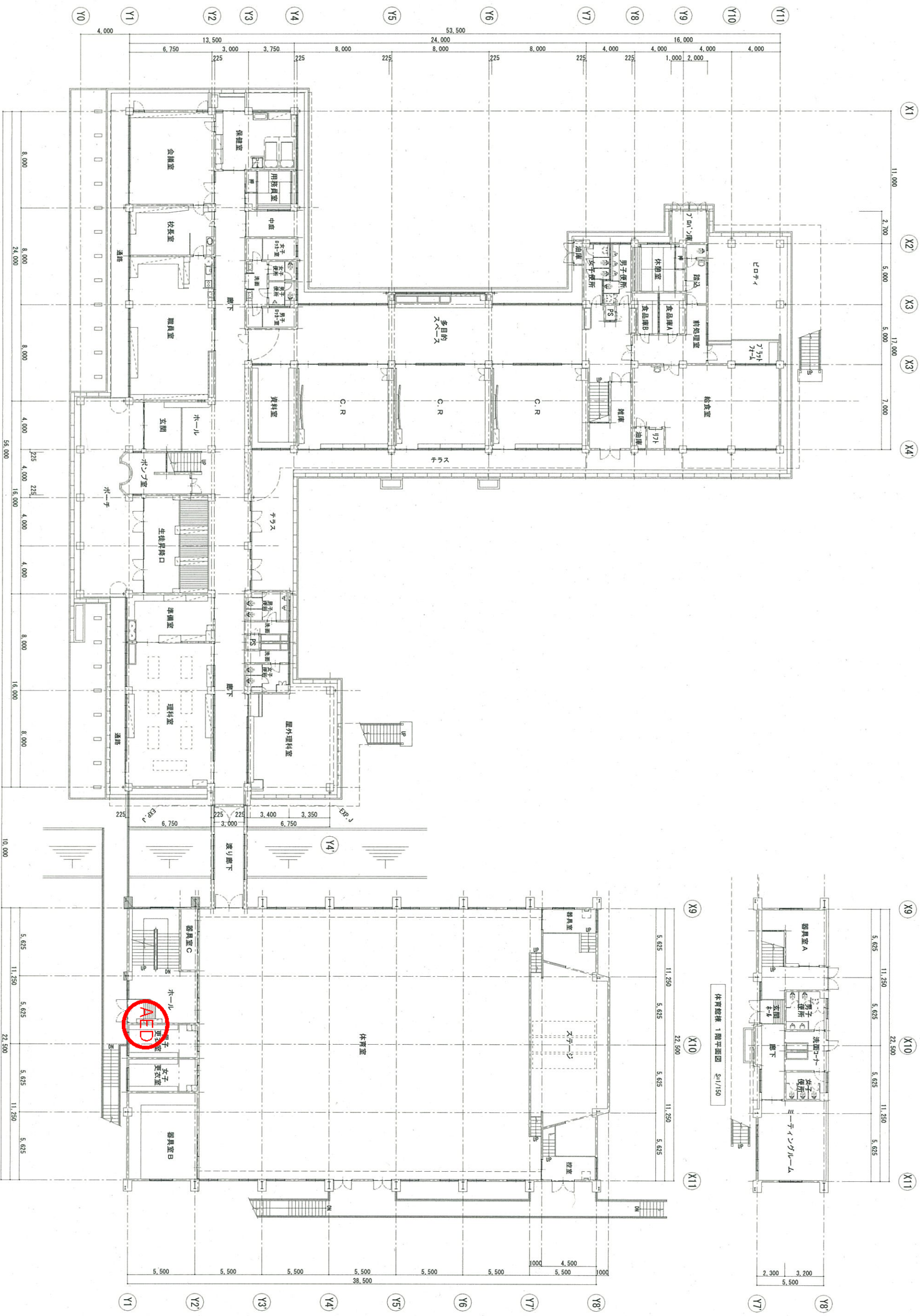
校舎棟 1階平面図 S=1/150
