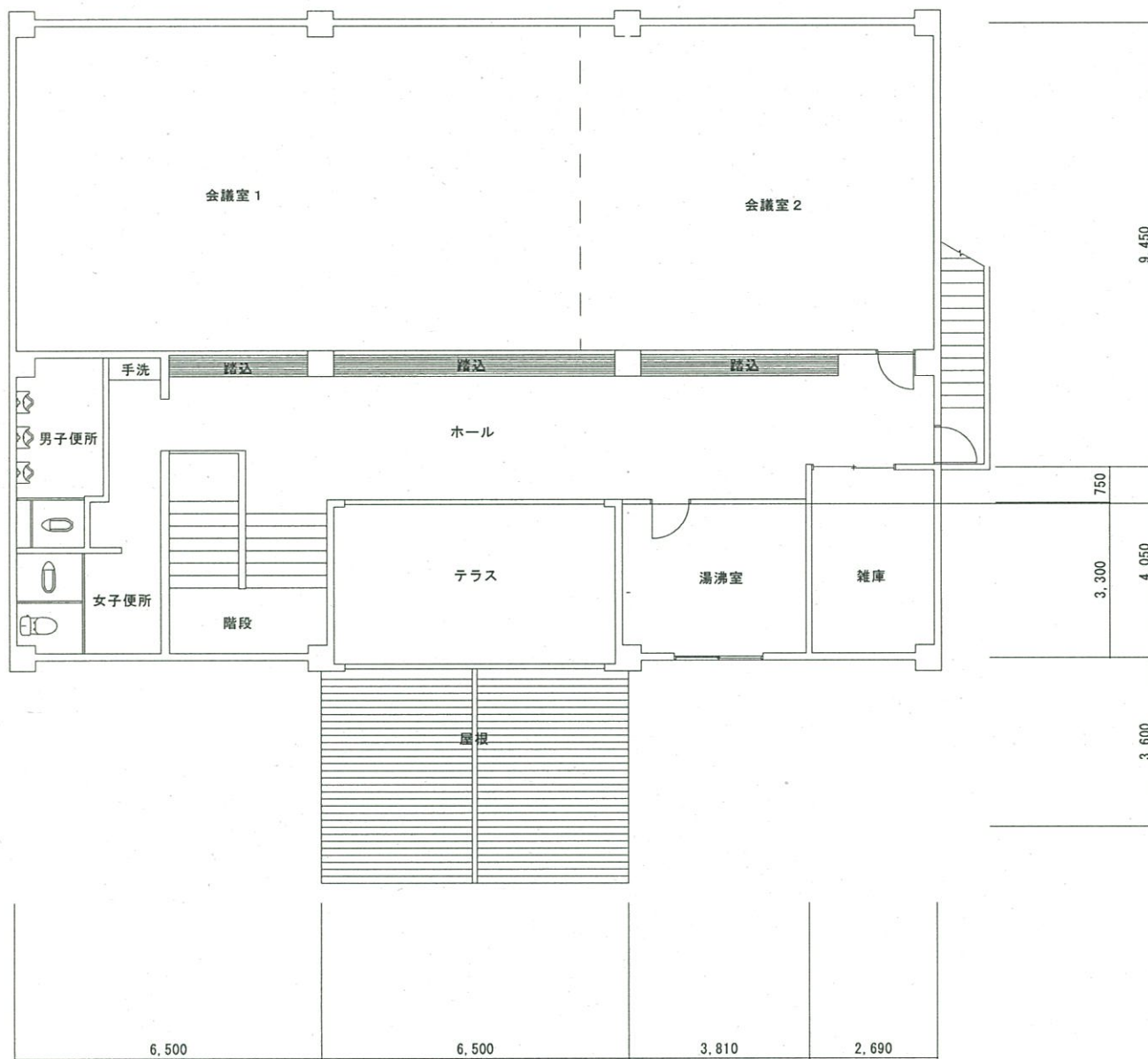
2階平面図
