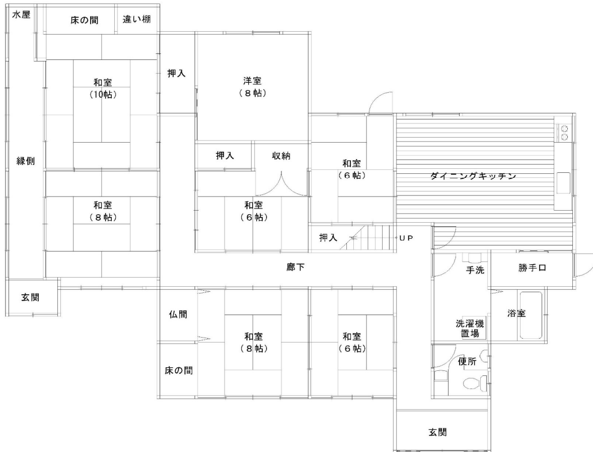
1階平面図
