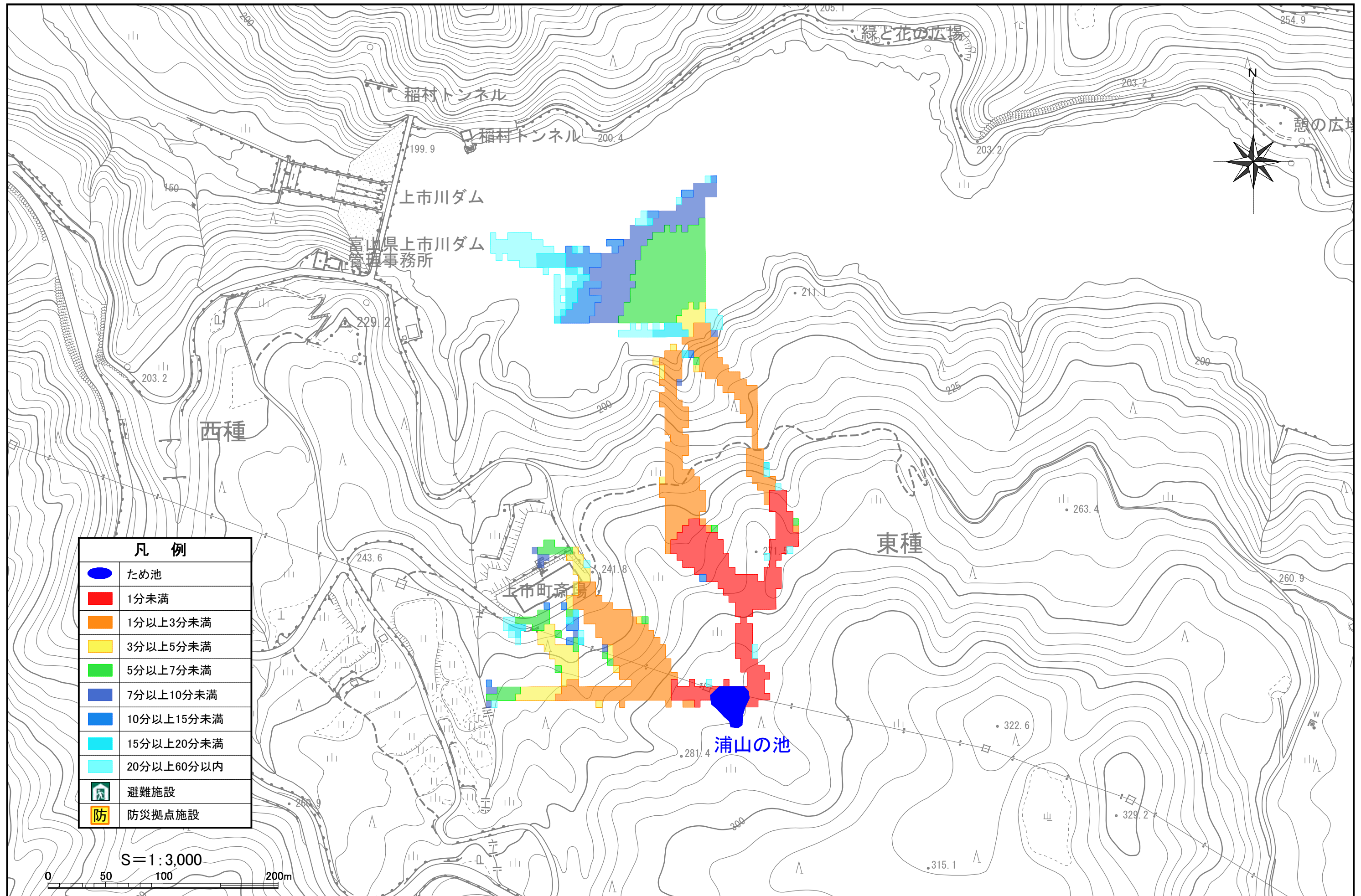
上市町 ため池浸水想定範囲図(氾濫解析結果-到達時間) 【浦山の池】
