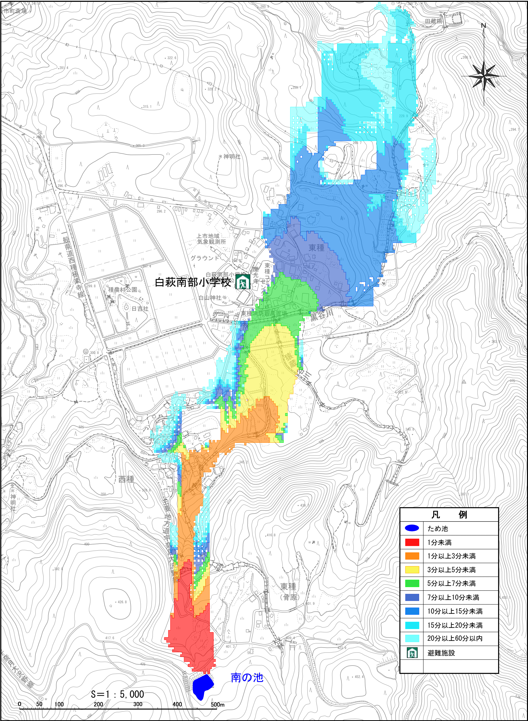
上市町 ため池浸水想定範囲図（氾濫解析結果-到達時間） 【南の池】
