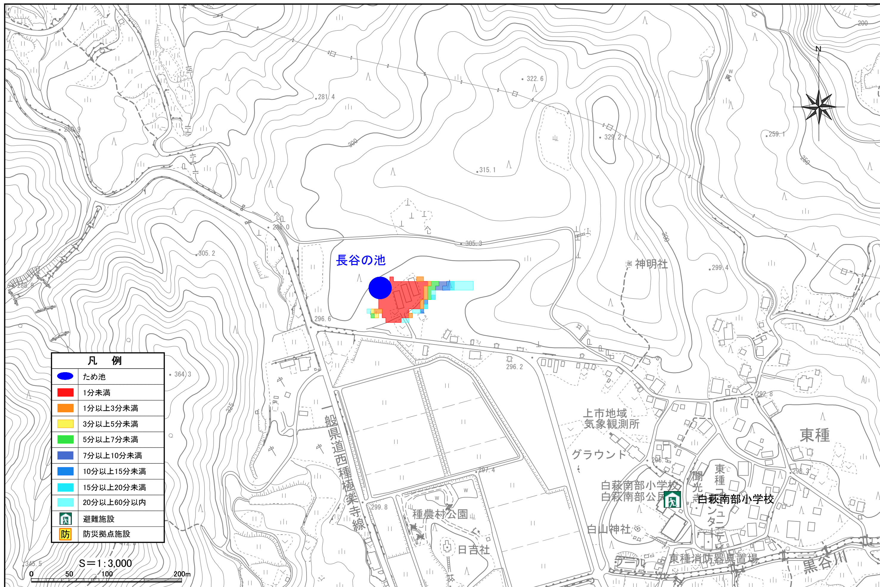
上市町 ため池浸水想定範囲図(氾濫解析結果-到達時間) 【長谷の池】
