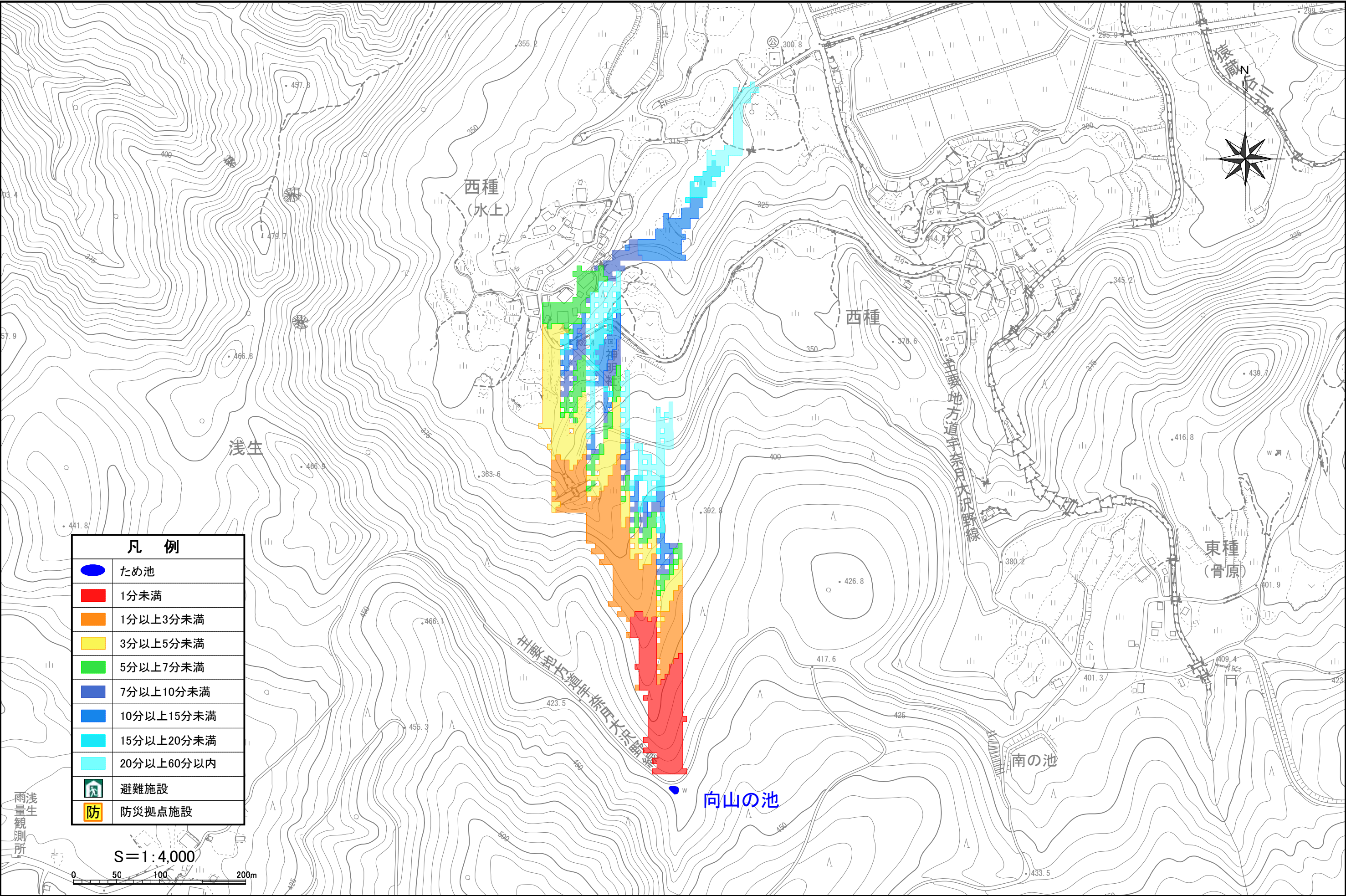
上市町 ため池浸水想定範囲図(氾濫解析結果-到達時間) 【向山の池】
