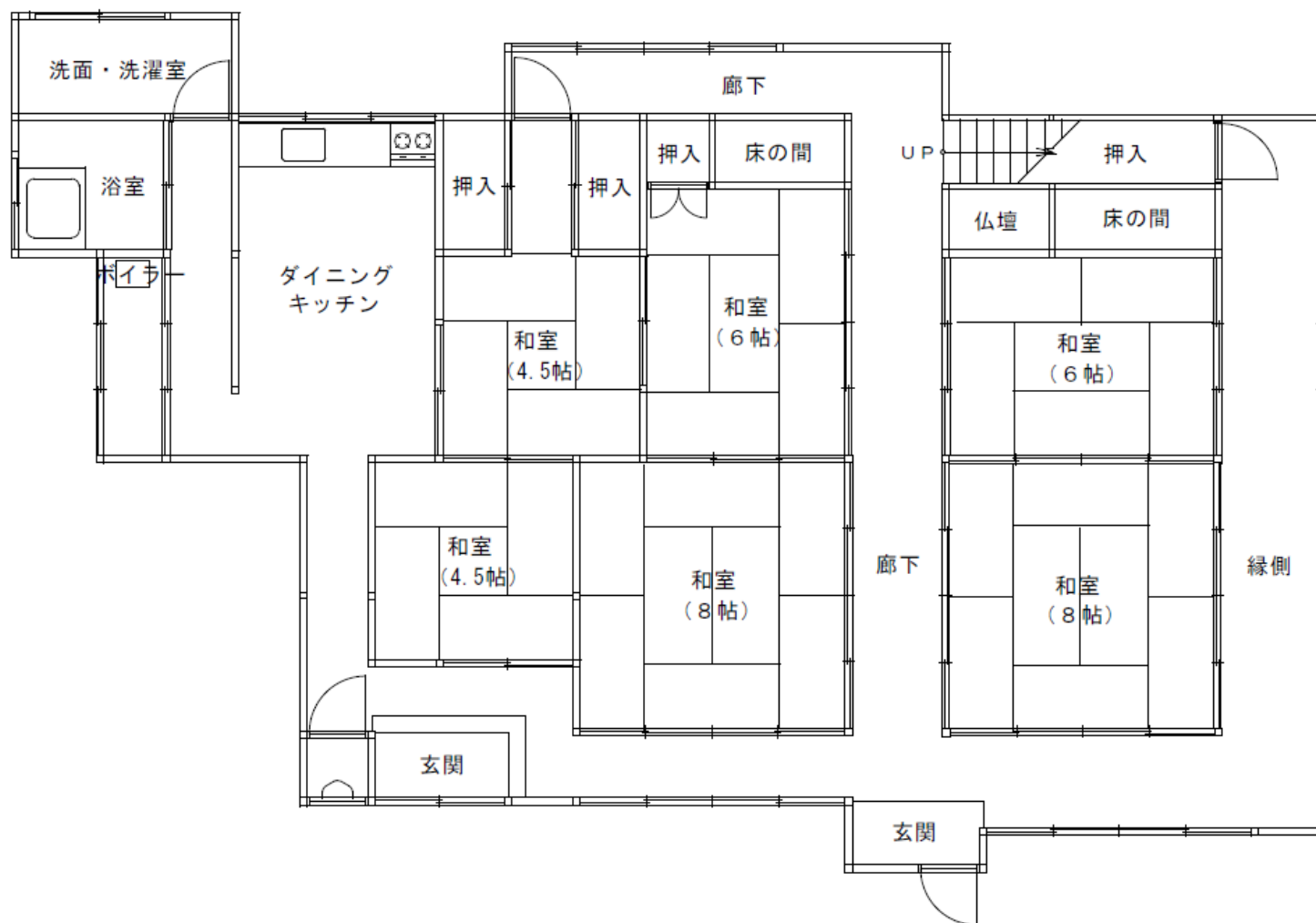
1 階平面図
