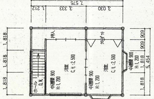
2階平面図 S:1/100
